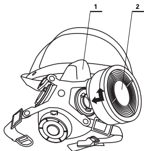
Rys. 5 Układ do ochrony przed szkodliwymi gazami i parami.
