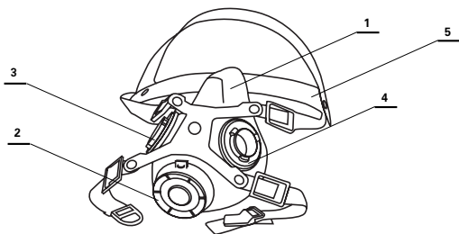
Rys. 1 Półmaska SECURA 2000
