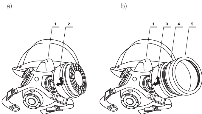
Rys. 6 Układy funkcjonalne do ochrony układu oddechowego przed szkodliwymi aerozolami i gazami.
