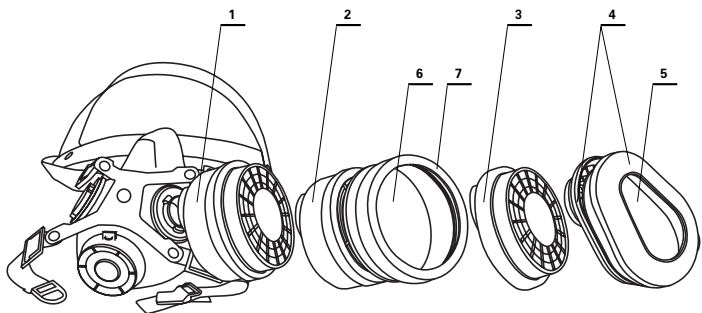
Rys. 00 Półmaska SECURA 2000 i elementy oczyszczające przeznaczone do kompletowania odpowiednich układów użytkowych.
